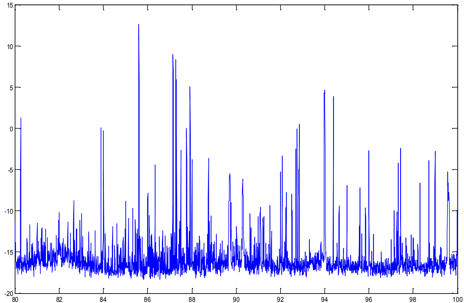
Figure 8: Spectre du bruit sur la banc (dB – MHz) FMO_Kourou35
