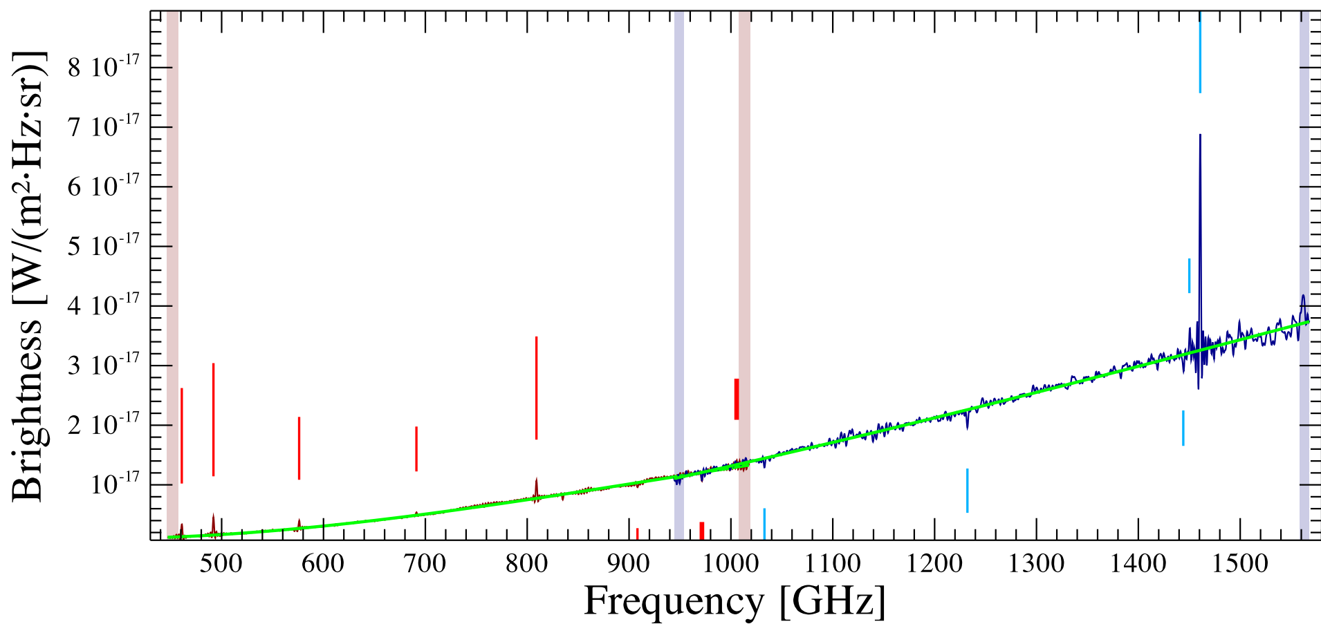
OH30.7+0.4 Observation ID 1342268309; (8/5)
