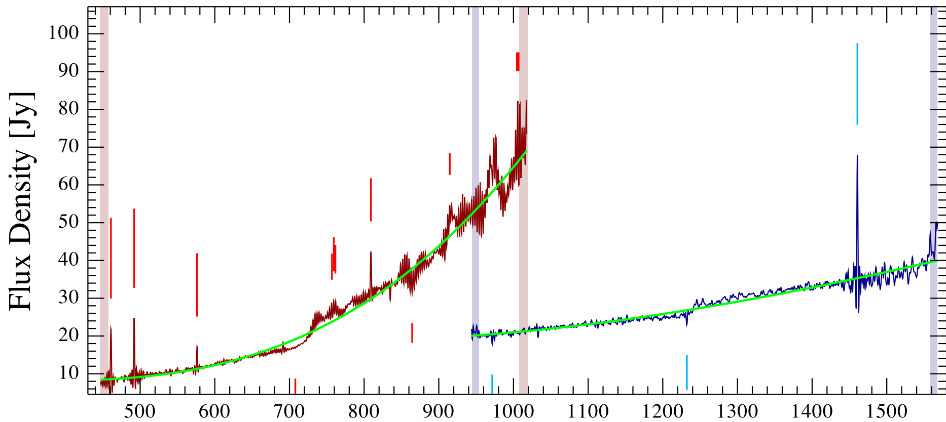
OH30.7+0.4 Observation ID 1342268309; (8/5)
