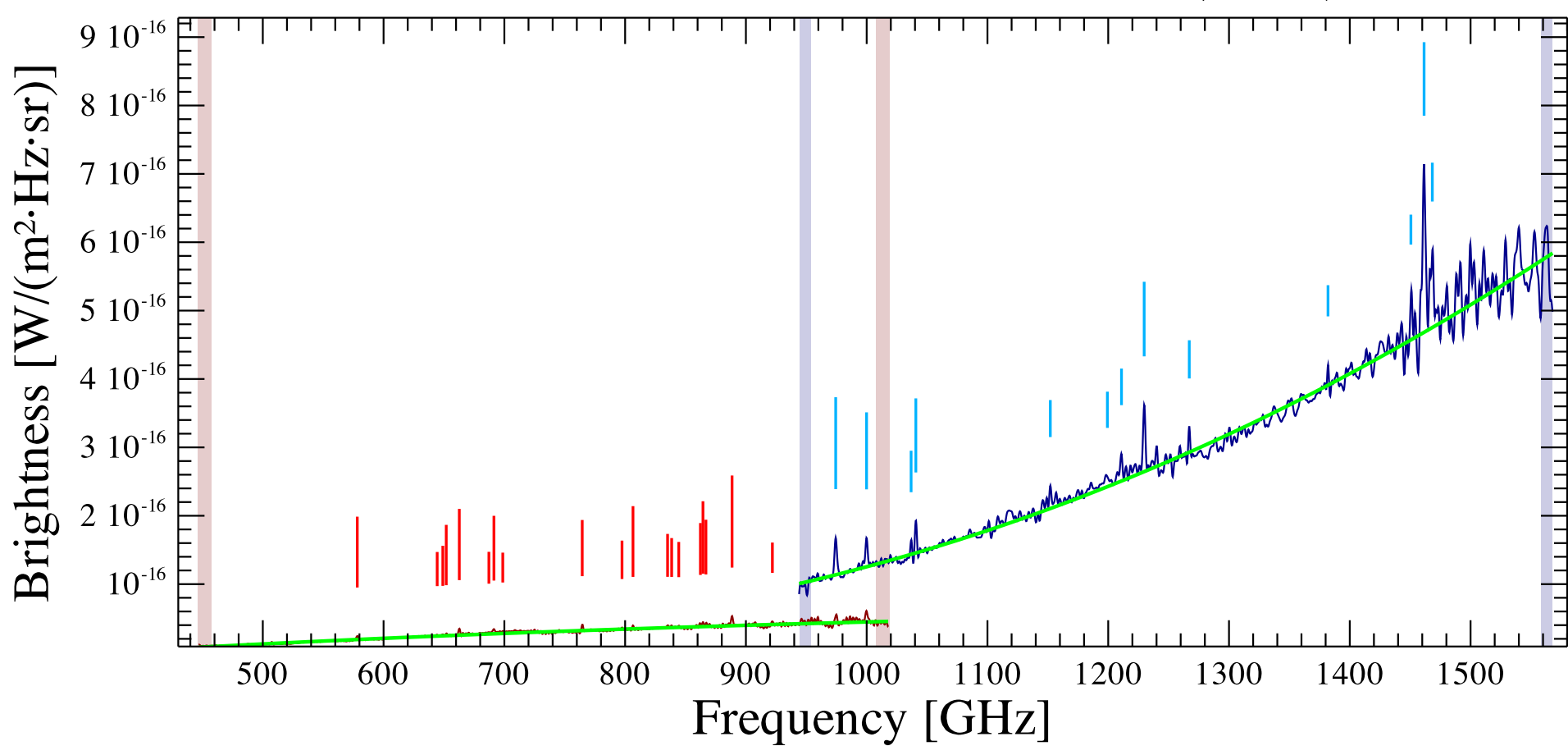
Eta Car Observation ID 1342228699; (22/13)
