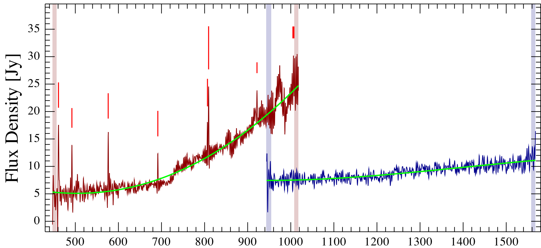
EL29_int Observation ID 1342204896; (7/0)
