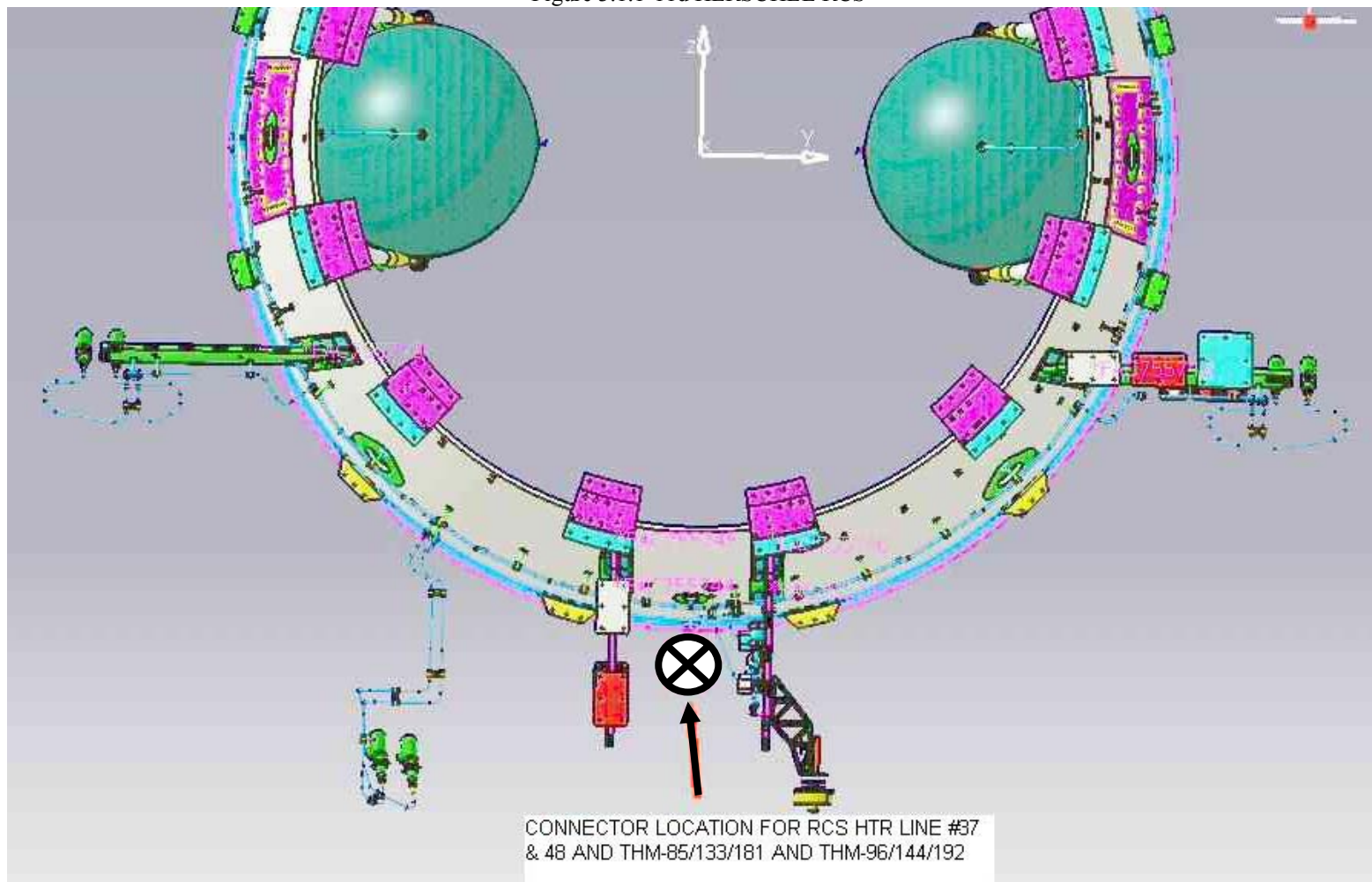
Figure 3.1.1-11d HERSCHEL RCS
