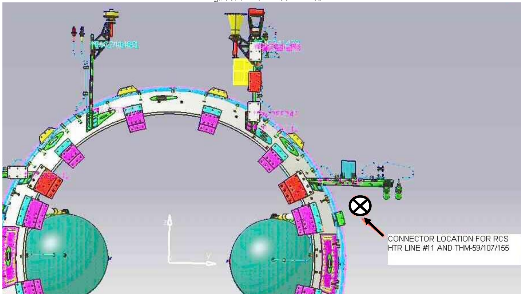
Figure 3.1.1-11b HERSCHEL RCS
