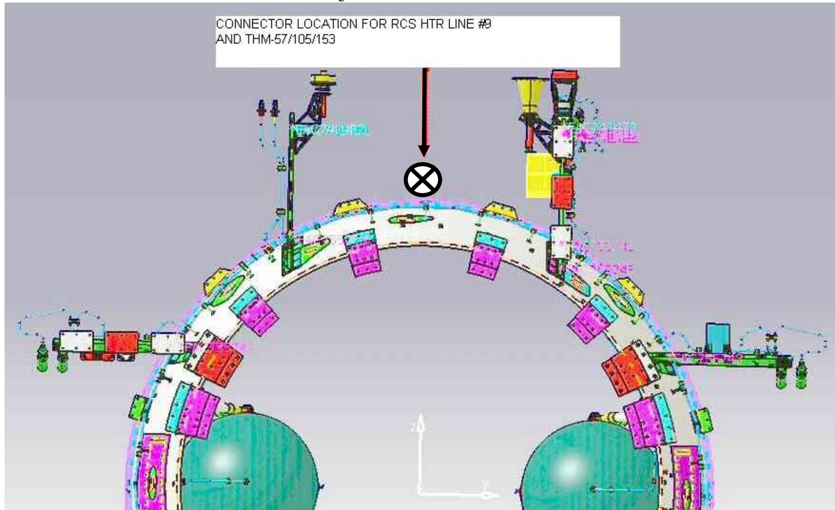
Figure 3.1.1-11a HERSCHEL RCS
