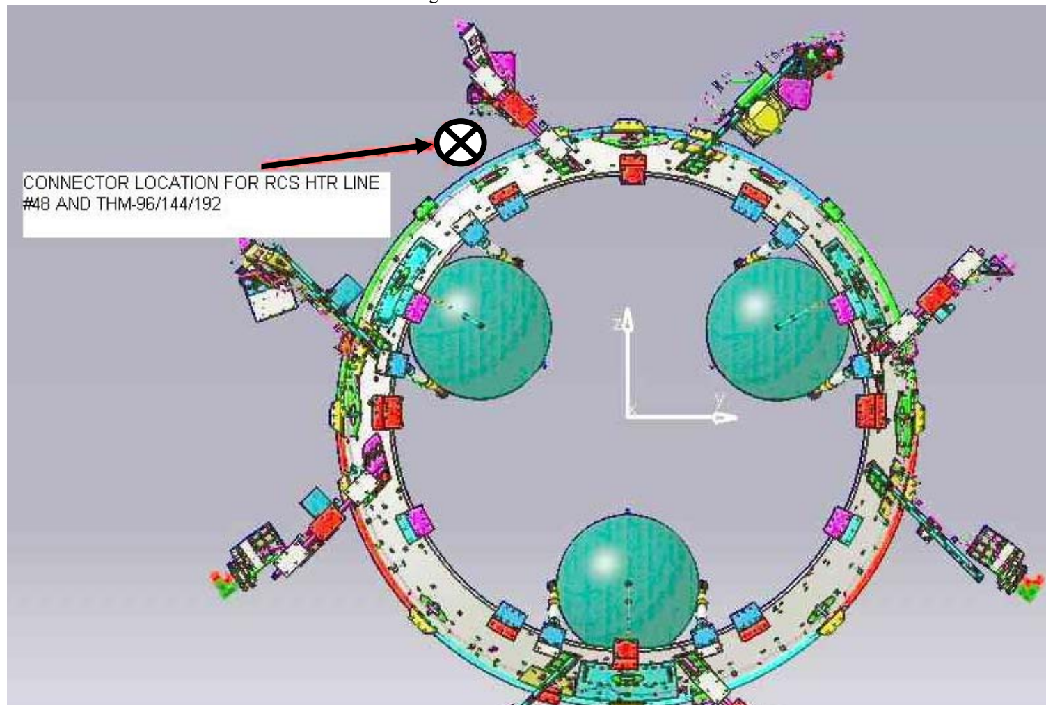
Figure 3.1.2-14e PLANCK RCS
