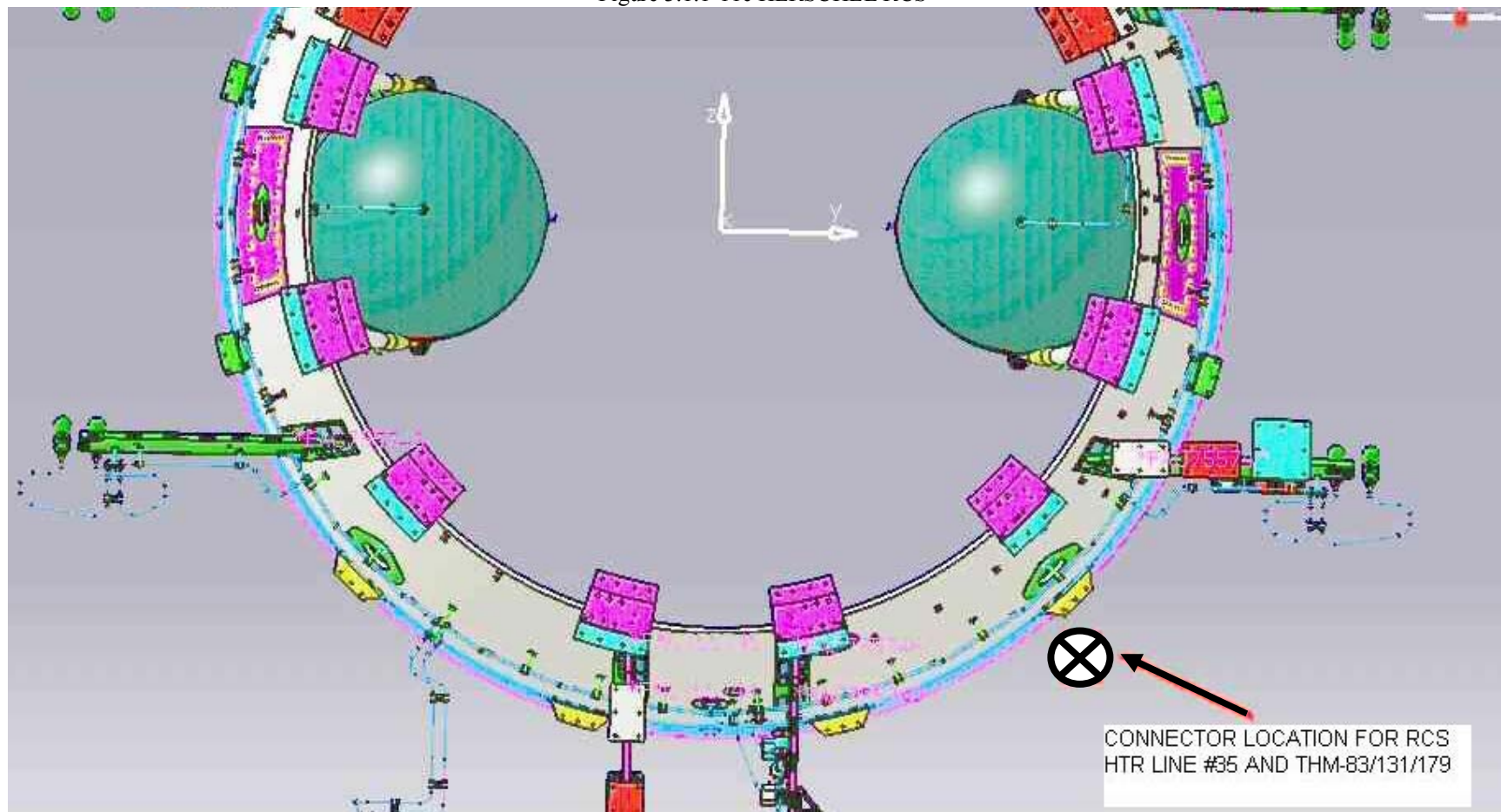
Figure 3.1.1-11c HERSCHEL RCS
