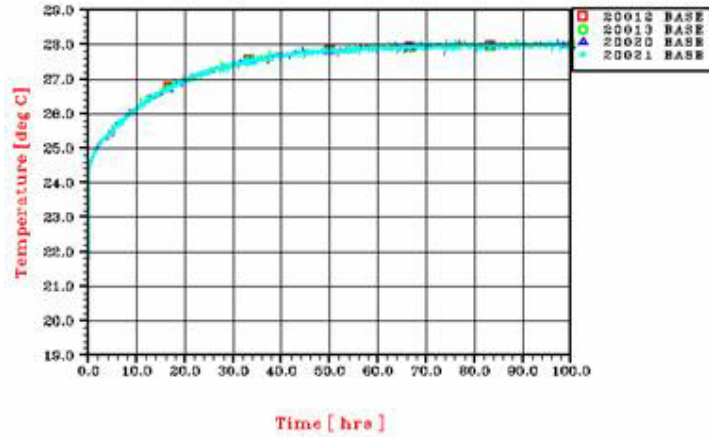
HERSCHEL HOT CASE C EOL 2STR ON STR2
