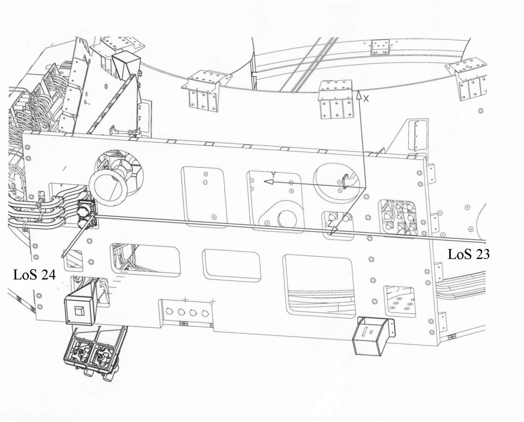
Herschel SVM AAD LoS definition.
