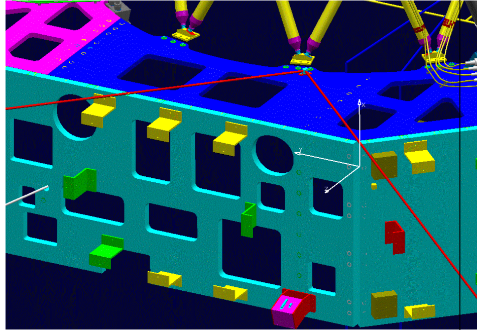
MRC4 (AC1) LOS
