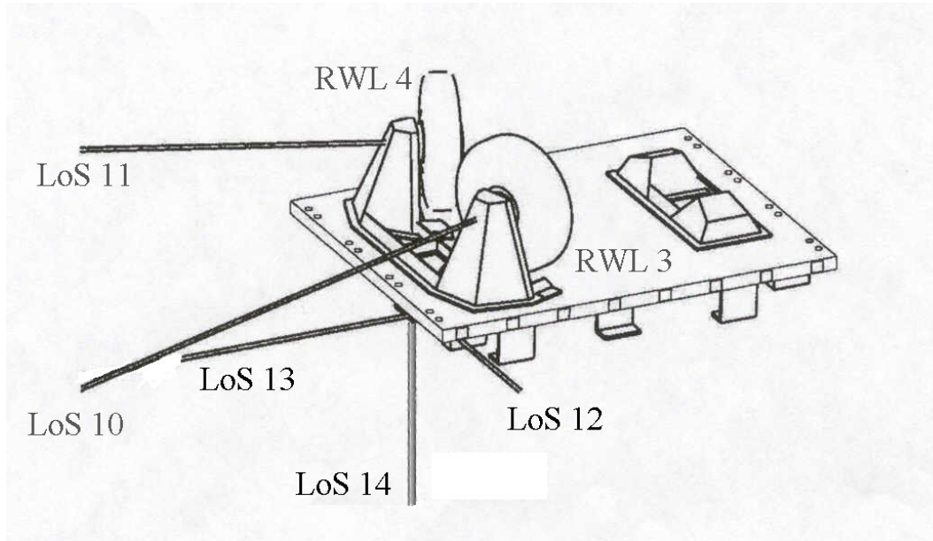
Herschel RWL 3 & 4 LoS definition. - -Y+Z panel
