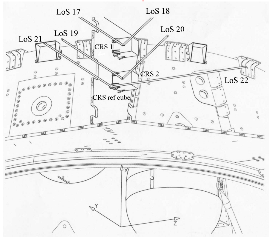
Herschel CRS 1&2 +ref cube LoS definition.
