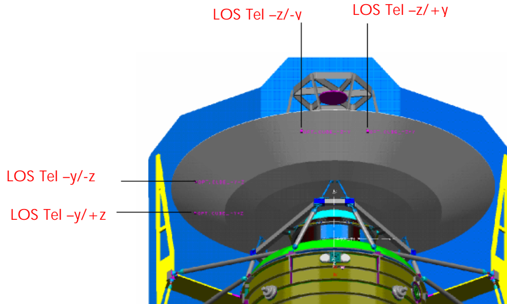
Telescope LOS description
