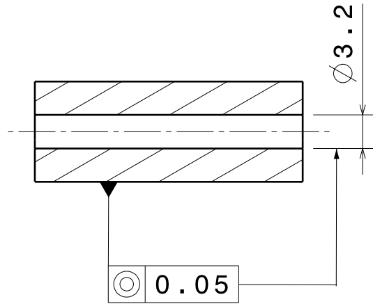
Coupe A-A
