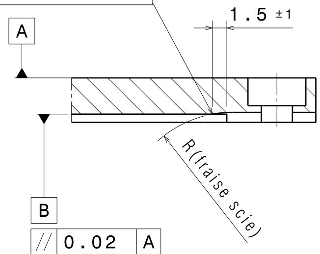
Coupe B-B Echelle : 3:1
